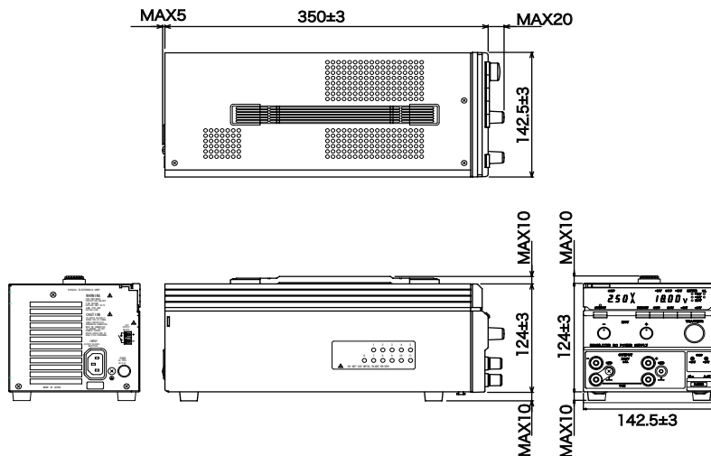
図 6-1 PMM18-2.5DU 外形寸法図 単位 : mm
