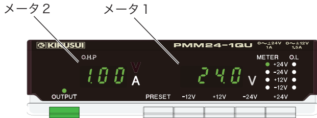
図 5-7 PMM24-1QU メータ表示 (メータ 1, メータ 2)
