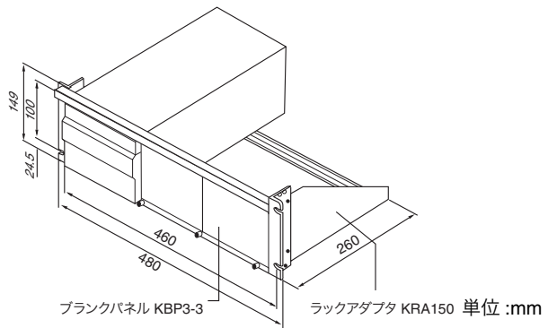
図 1-2 ラックマウントオプション取り付け例 (ミリラック)
