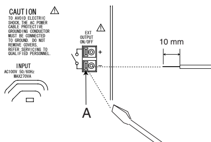
図 4-10 EXT OUTPUT ON/OFF 端子への接続
