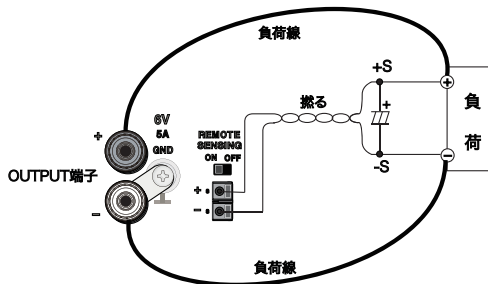
図 4-6 センシング線の接続
