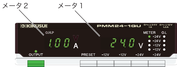
図 5-8 PMM24-1QU メータ表示 (メータ 1, メータ 2)
