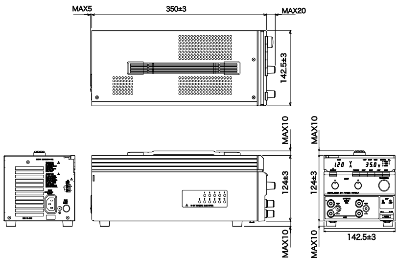
图 6-2 PMM35-1.2DU 外形寸法图 单位：mm
