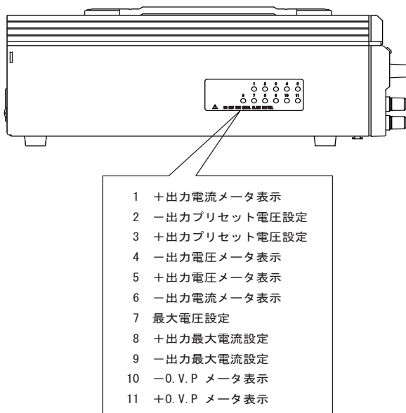
図 5-2 PMM18-2.5DU, PMM35-1.2DU 校正用可変抵抗器
