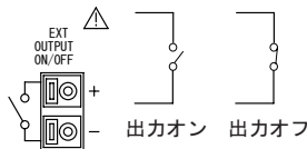
図 4-9 EXT OUTPUT ON/OFF コネクタ
