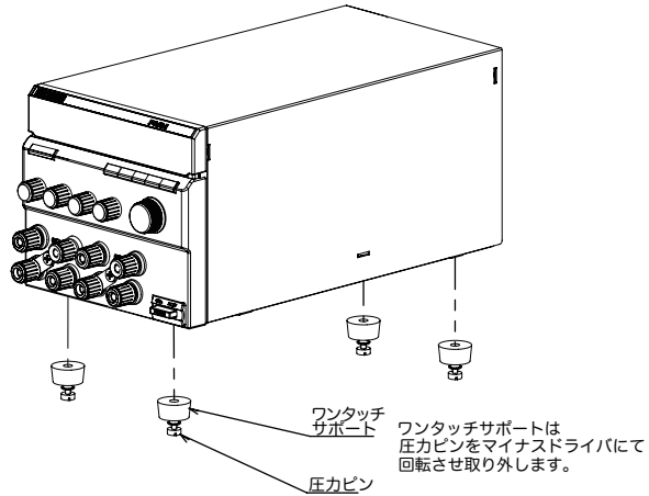
図 2-2 ゴム足の取り外し方
