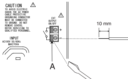
図 4-13 EXT OUTPUT ON/OFF 端子への接続
