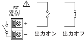
図 4-12 EXT OUTPUT ON/OFF コネクタ
