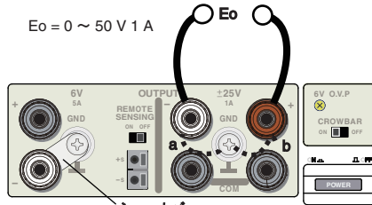
図 4-7 PMM25-1TR の直列運転例
