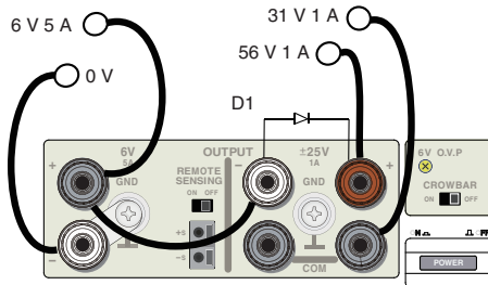
図 4-8 PMM25-1TR の直列接続例（マイナス接地の例）
