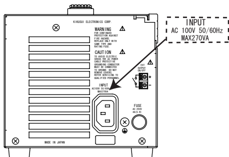
図 2-3 公称入力定格の確認
