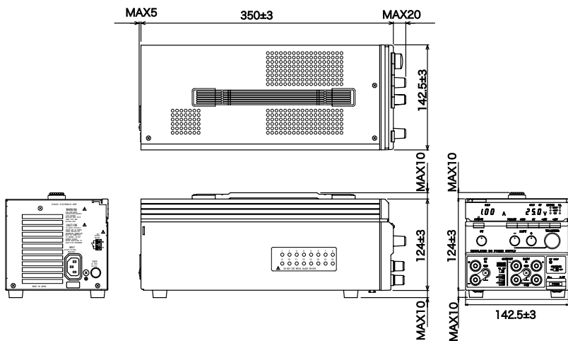
图 6-3 PMM25-1TR 外形寸法图 单位：mm
