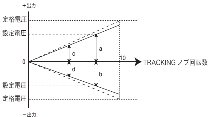
図 4-1 電圧設定とトラッキング出力
