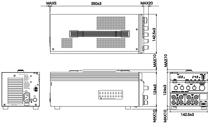
图 6-4 PMM24-1QU 外形寸法图 单位：mm
