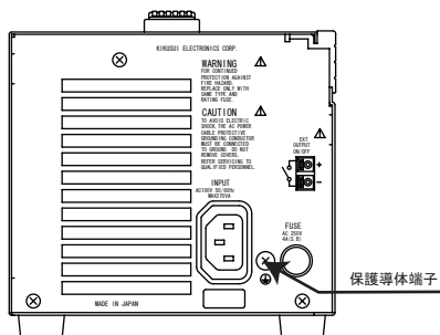
図 2-4 接地 (保護導体端子) の確認
