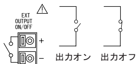
図 4-3 EXT OUTPUT ON/OFF コネクタ
