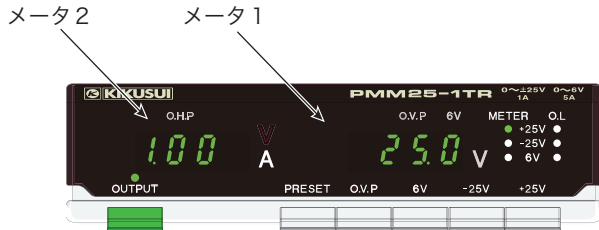
図 5-5 PMM25-1TR メータ表示 (メータ 1, メータ 2)
