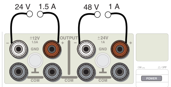
図 4-11 PMM24-1QU の直列運転例
