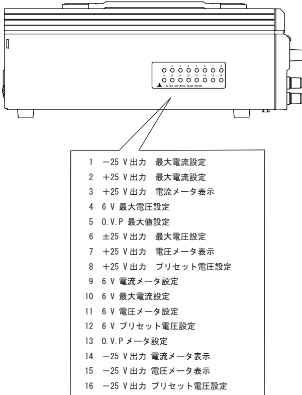
図 5-4 PMM25-1TR 校正用可変抵抗器
