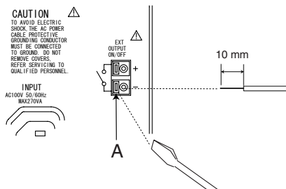
図 4-4 EXT OUTPUT ON/OFF 端子への接続
