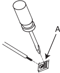
図 4-5 センシング端子への接続
