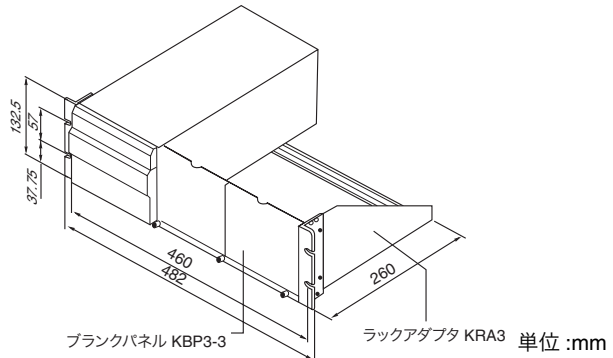
図 1-1 ラックマウントオプション取り付け例 (インチラック)
