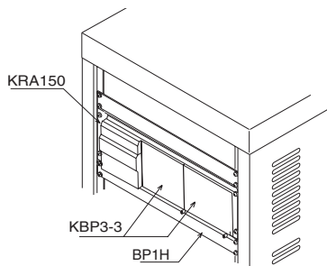
図 1-3 ラック組み込み例
